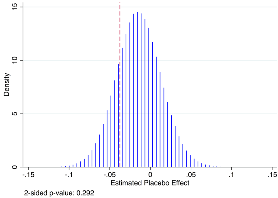
Panel A: All Placebo Estimates
