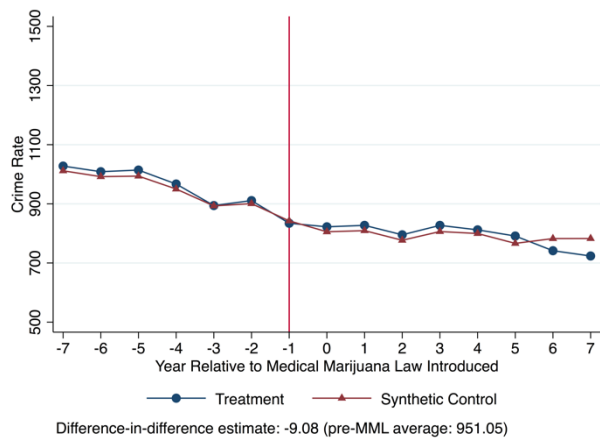
Panel A: Burglary
