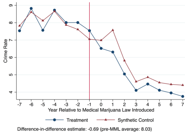
Panel A: Murder
